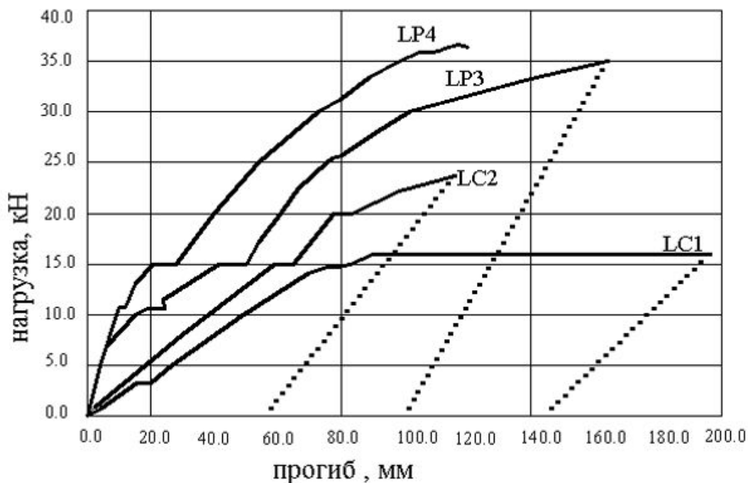
Рисунок 7 – Результаты испытаний балок
