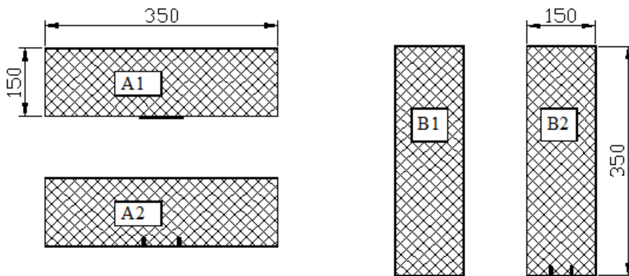
Рисунок 8 – Усиление железобетонных колонн установкой КМФУ в пазы
