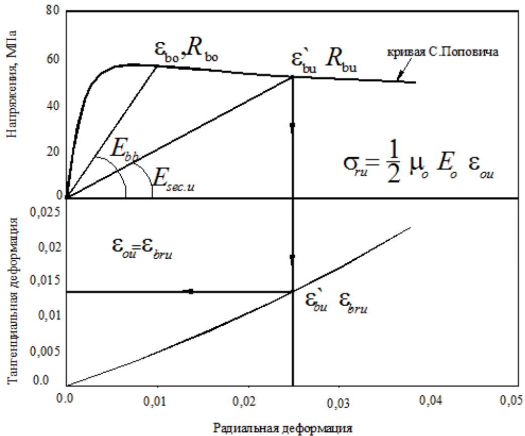
Рисунок 37 – Определение предельных сжимающих напряжений и деформаций
