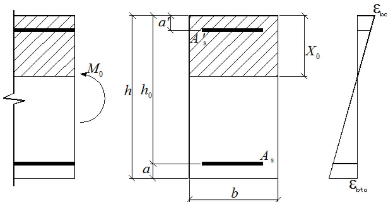
Рисунок 13 – Начальное напряженно-деформированное состояние элемента перед усилением
