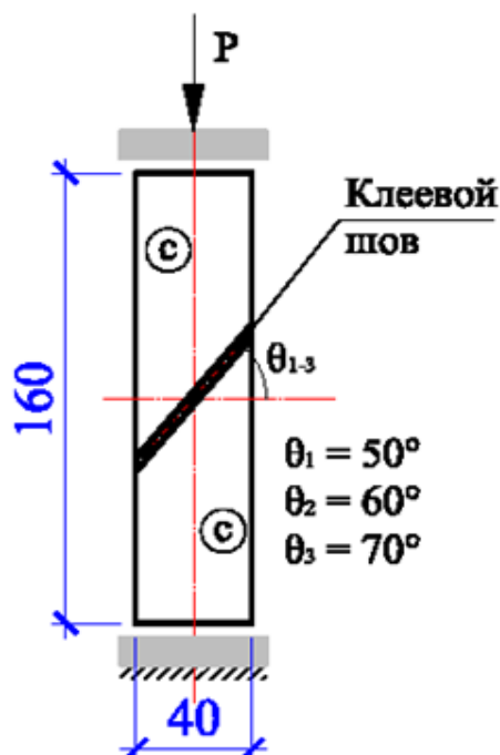
Рисунок 42 – Схема испытаний клеевого соединения сталь/сталь срезающим разрушением (косой сдвиг при осевом сжатии, образец-призма 40х40х160 мм)
