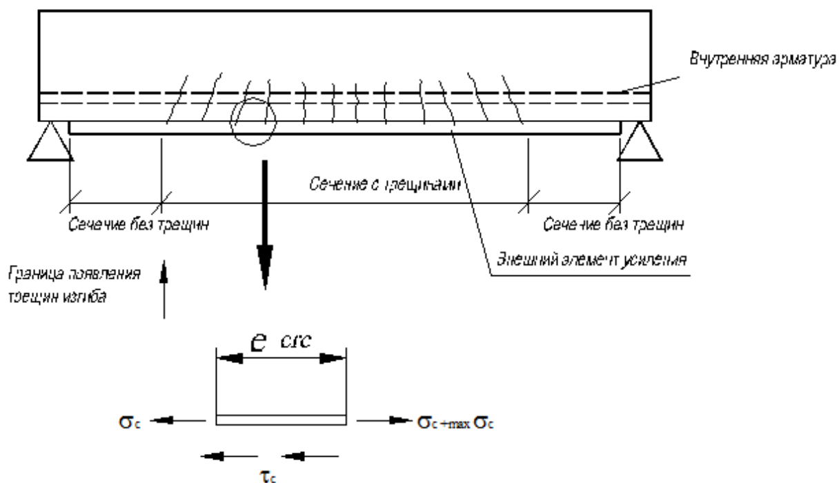
Рисунок 27 – Анализ появления отслоения при изгибе между трещинами
