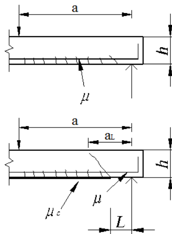
Рисунок 29 – Концепция потери сцепления материала усиления с железобетонной конструкцией от действия сдвиговых усилий: \mu_c – коэффициент армирования конструкции композитным материалом; \mu – коэффициент армирования конструкции стальной арматурой; h – высота сечения конструкции; L – расстояние от опоры до ленты композитного материала; a_L – расстояние от опоры до верхней границы крайней к опоре наклонной трещины; a – расстояние от точки приложения силы до опоры.
