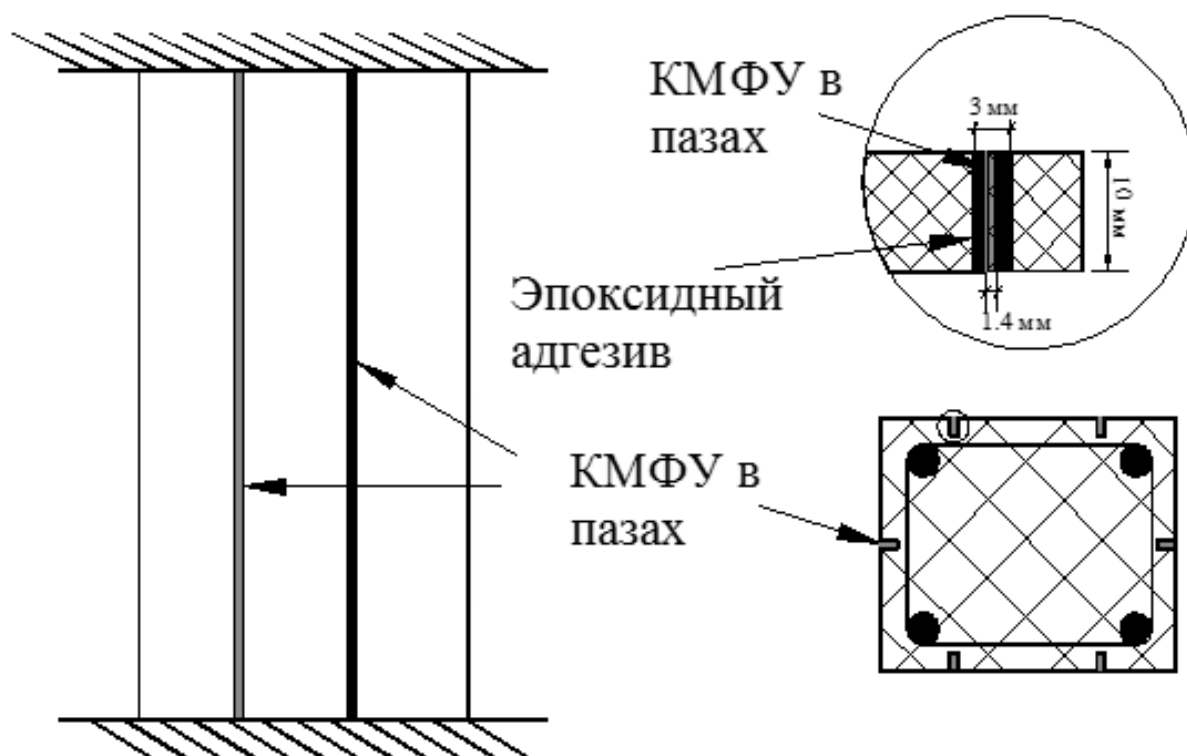
Рисунок 8 – Усиление железобетонных колонн установкой КМФУ в пазы
