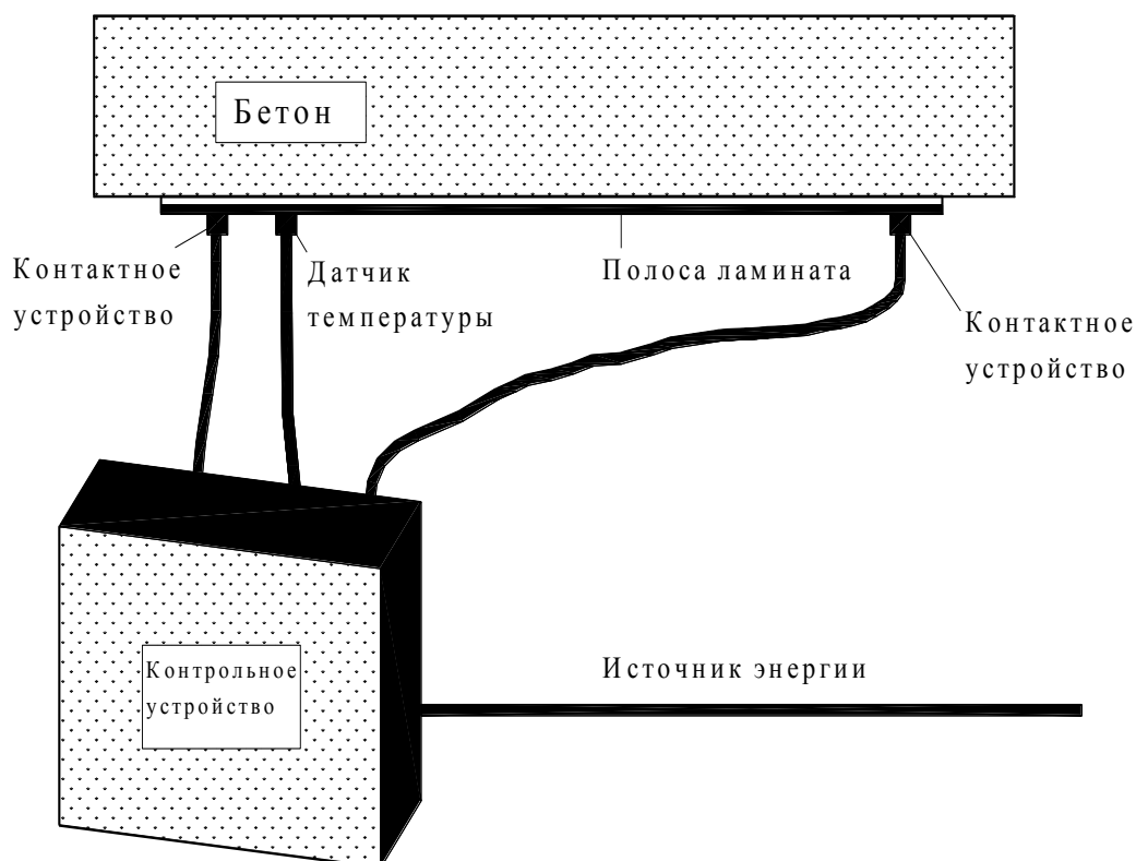
Рисунок 4 – Устройство нагрева при приклеивании ламината
