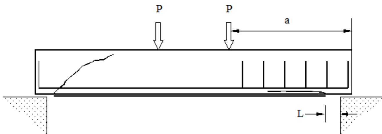
Рисунок 23 – Характер разрушения на конце полосы КМФ
