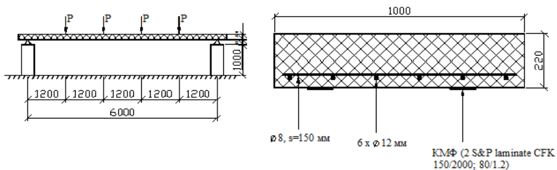
Рисунок 6 – Схема проведения испытаний
