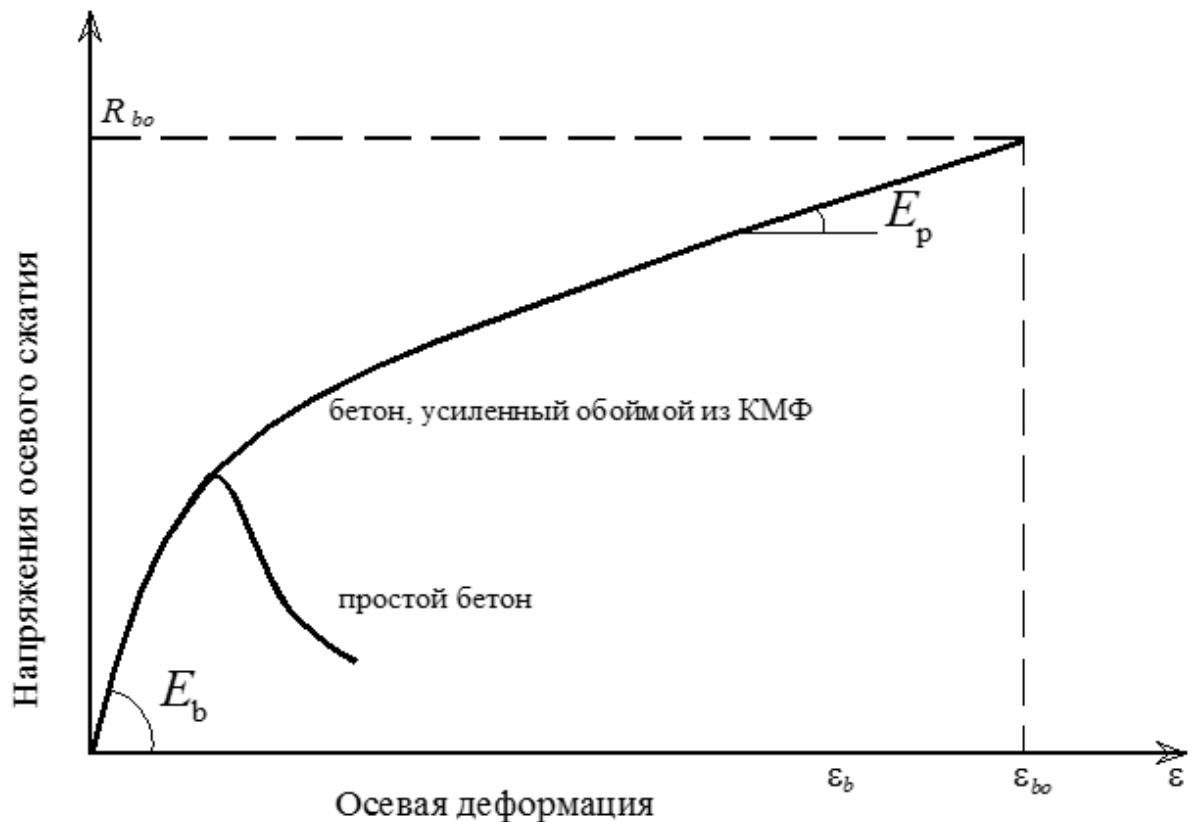
Рисунок 32 – Идеализированная диаграмма « \sigma - \epsilon » для бетона, усиленного обоймой из КМФ. E_b и E_p – Начальный и текущий модули деформации бетона, МПа
