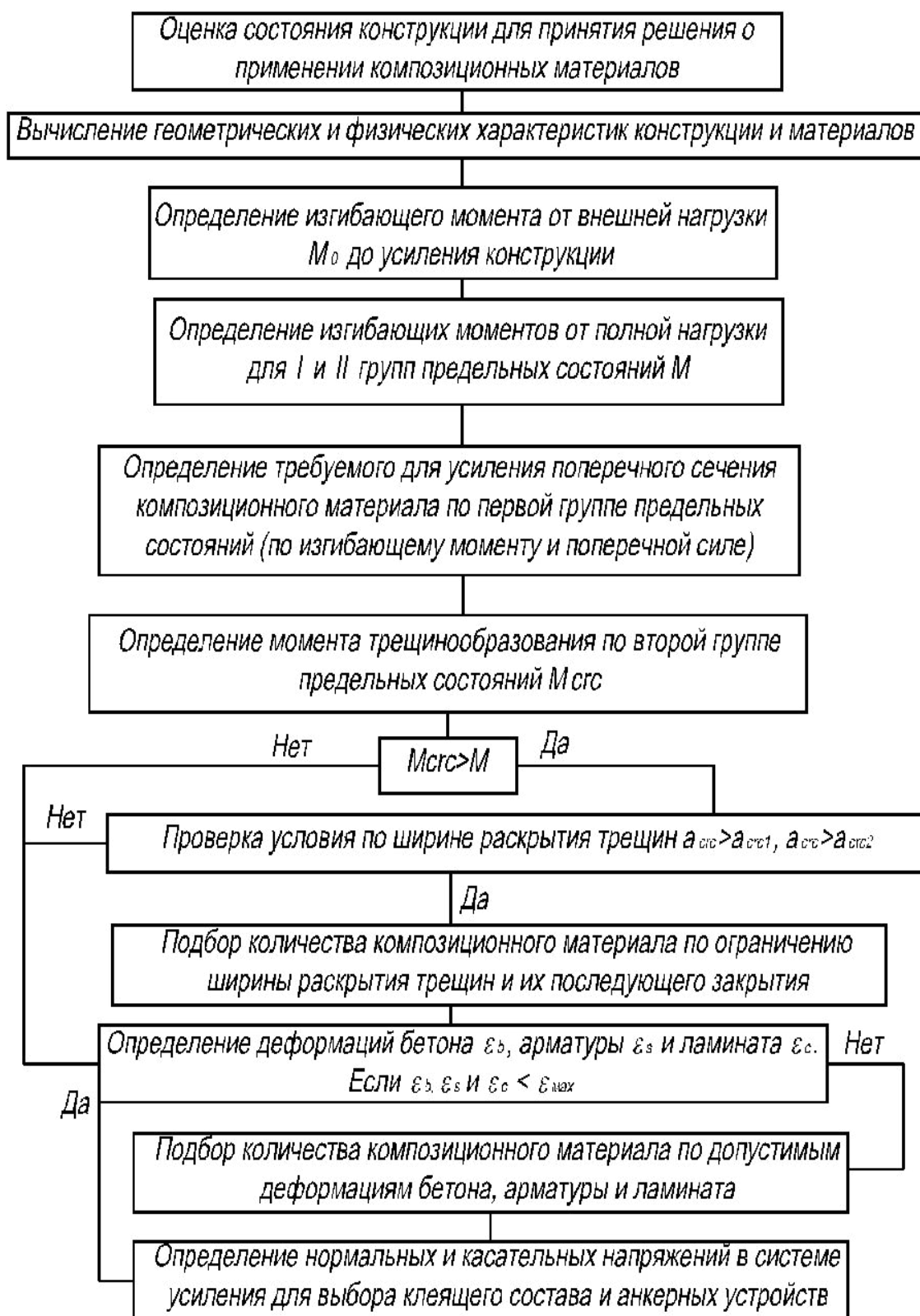
Рисунок 19 – Блок-схема проектирования усиления железобетонных конструкций композитными материалами
