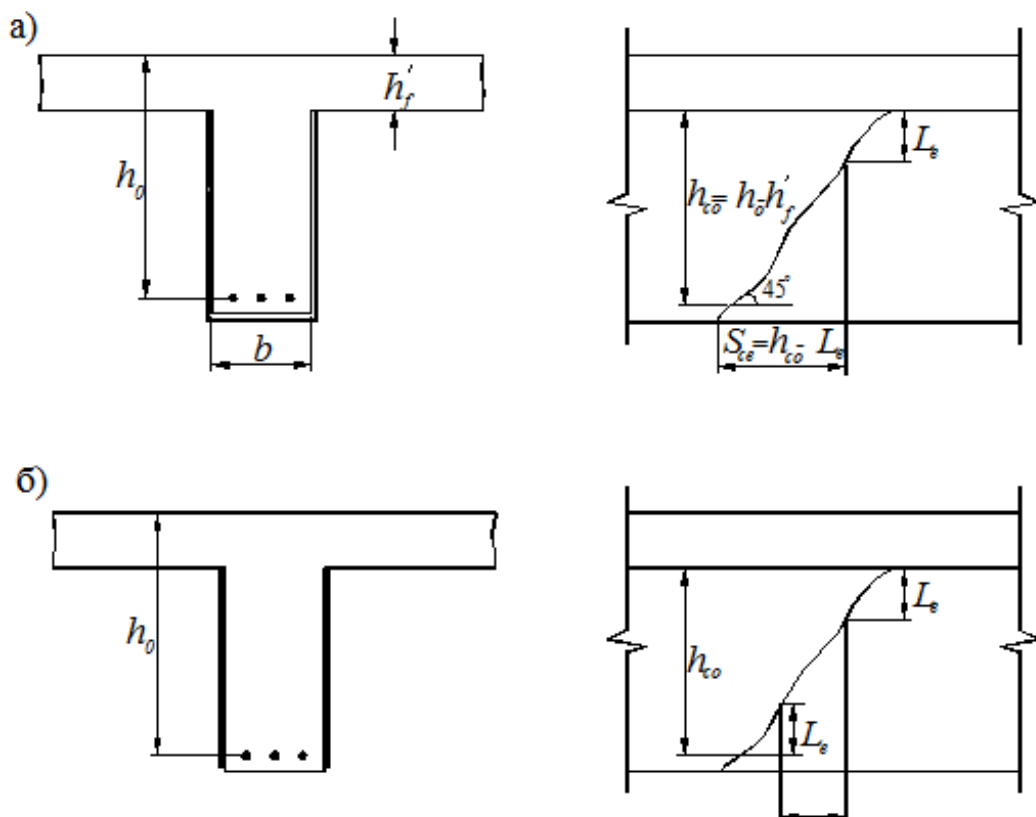
Рисунок 18 – Схемы к определению эффективной ширины полосы КМФ:
