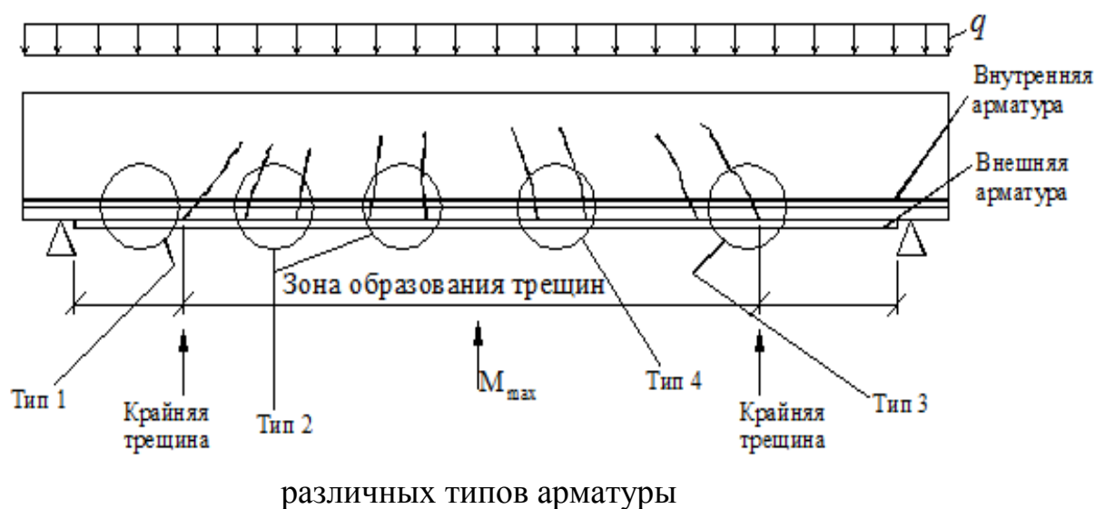
Рисунок 22 – Типы разрушения железобетонной конструкции, усиленной КМФУ
