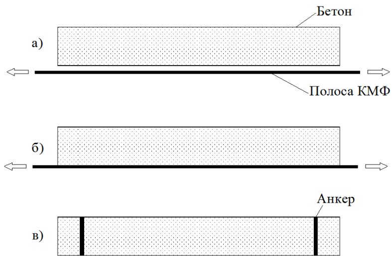
Рисунок 5 – Схема применения преднапряженных полос КМФ:
