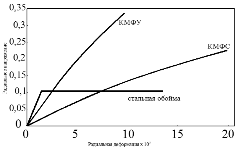
Рисунок 30 – Сравнительные графики усиления обоями из стали и композитных материалов
