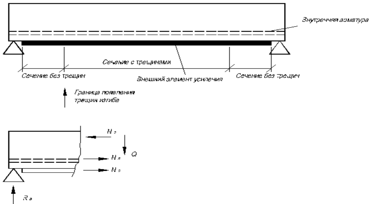
Рисунок 25 – Разделение анкеровки на границе возникновения трещин:
