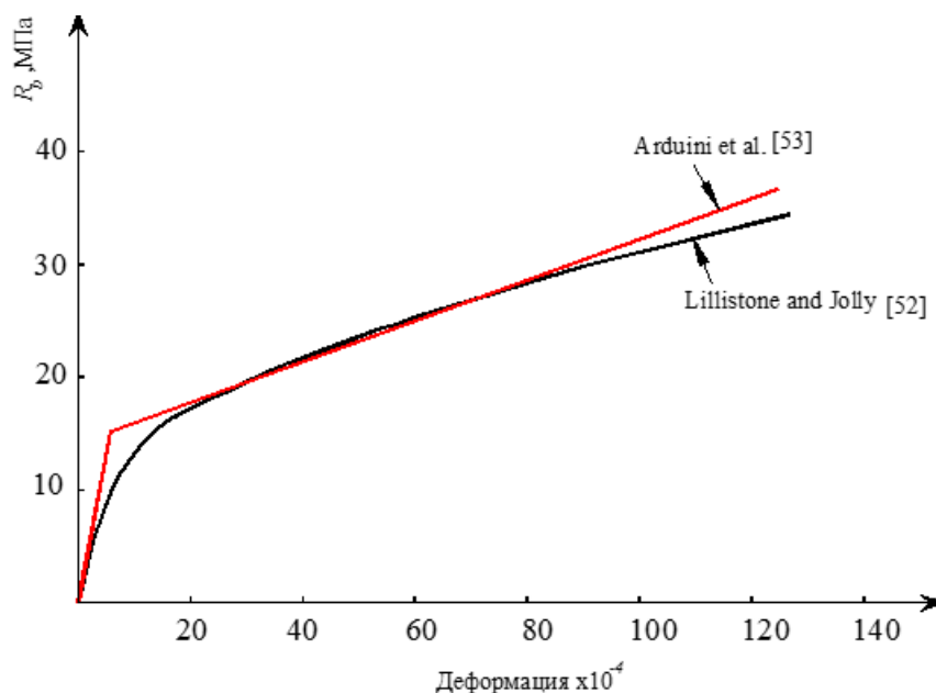
Рисунок 34 – Сравнительные диаграммы «напряжение-деформация»
