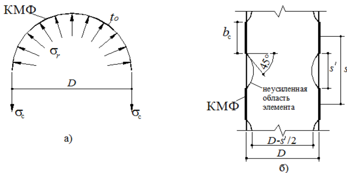
Рисунок 36 – Радиальное давление, вызываемое обоймой из КМФ, а) полное усиление по всей длине колонны; б) частичное усиление по длине колонны, где D – диаметр колонны; b_c – ширина ленты композитного материала; t_0 – толщина обоймы из композитного материала; \sigma_r – радиальные напряжения в конструкции, вызываемые обоймой из КМФ; s – расстояние между осями лент усиления КМФ; s' – расстояние между лентами усиления КМФ; \sigma_c – расчетные растягивающие напряжения в КМФ
