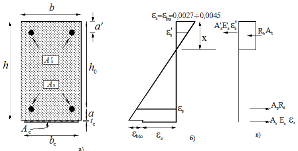
Рисунок 14 – Напряженно-деформированное состояние усиленного КМФ железобетонного элемента при изгибе: а) поперечное сечение; б) распределение деформаций; в) распределение сил
